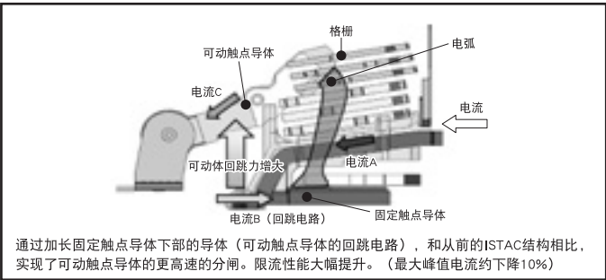
分断容量提升示例：250A 壳架 NF-H
