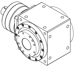
RT-AS 系列 ( 齒輪比 1/2~1/5 ) : RF 中空旋轉 法蘭型式尺寸圖
