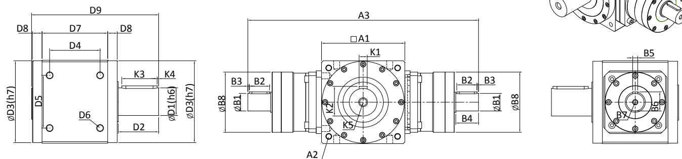
RT-(2AX-P) 系列 ( 齒輪比 1/2 ~ 1/5 ) : 2AX-P 型 式尺寸圖
