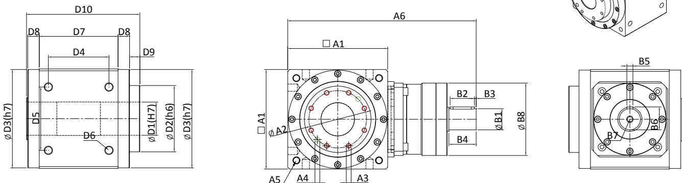
RT-AS 系列 ( 齒輪比 1/2~1/5 ) : RF 中空旋轉 法蘭型式尺寸圖
