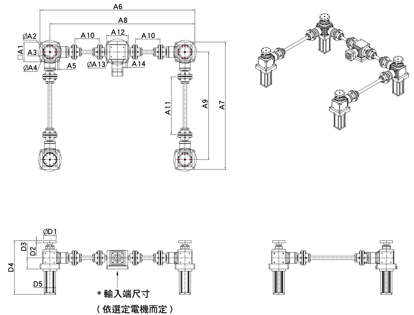
■ RB-G4U-AHT 系列：4 軸螺桿升降機活塞型式 - 尺寸圖
