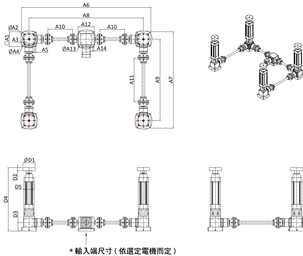
■ RB-G4U-A-JDT 系列：4 軸螺桿升降機電缸型式 - 尺寸圖
