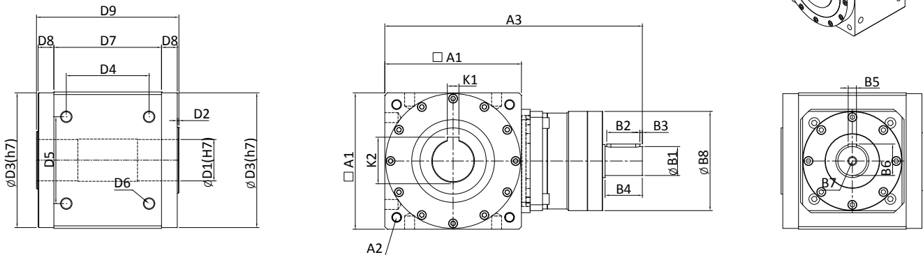
RT-A 系列 ( 齒輪比 1/1 ) : CR 中空軸帶鍵槽 型式尺寸圖
