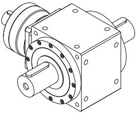
RT-A 系列 ( 齒輪比 1/1 ) : 2P 雙輸出軸型式尺寸圖
