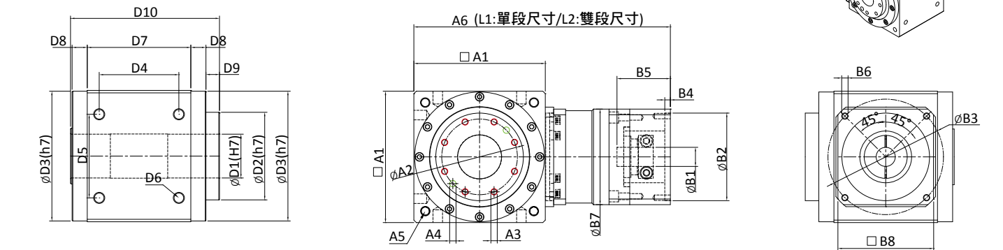
RXW-AS 系列：RF 中空旋轉盤型式 (L1/L2: 單段 / 雙段尺寸圖 )
